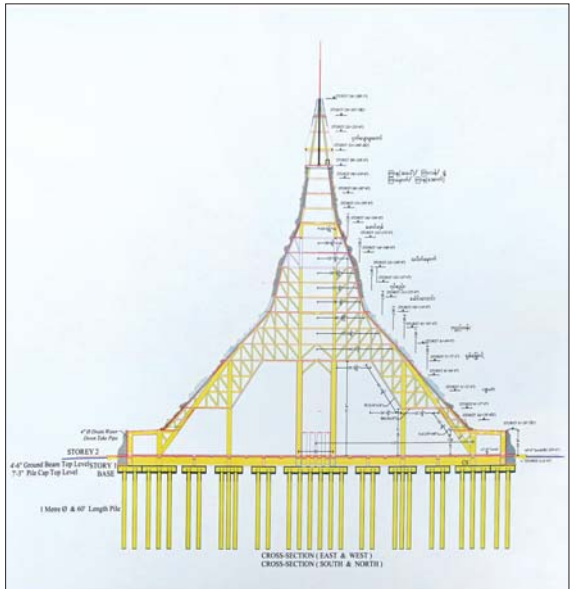
ဥပုတသန္တိစေတီတော်မြတ်ကြီး တည်ဆောက်ခဲ့ရာတွင် အချင်း ၁ မီတာရှိ Bored Pile ပေါင်း ၄၄၀ ပေါ်တွင် စနစ်တကျတွက်ချက်၍ အုတ်မြစ်ချတည်ဆောက်ခဲ့မှုကို တွေ့ရစဉ်။
