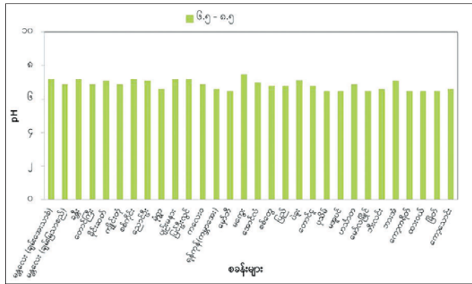
ပုံ(၂)၊ ၂၀၂၅ ခုနှစ် စက်တင်ဘာလအတွင်း ရွာသွန်းခဲသော မိုးရေ၏ pH တန်ဖိုးများပြပုံ။
