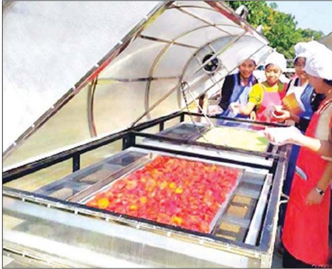
အသေးစားနေရာရောင်ခြည်သုံး အခြောက်ခံစက်ဖြင့် သီးနှံများအား အခြောက်ခံထားရှိစဉ်။
