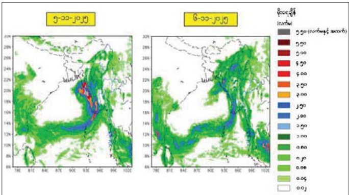
မိုးလေဝသနှင့်ဇလဗေဒဌာနကြားမှဦးစီးဌာန၊ WRF မော်ဒယ်၏ ၃၁-၁၀-၂၀၂၅ ရက်နေ့ မြန်မာစံတော်ချိန် ၀၆:၃၀ နာရီအချိန်ကို အခြေခံတွက်ထုတ်ထားသည့် ၅-၁၁-၂၀၂၅ ရက်နေ့မှ ၆-၁၁-၂၀၂၅ ရက်နေ့အထိ မိုးရွာသွန်းမှုခန့်မှန်းချက်ပြပုံ
